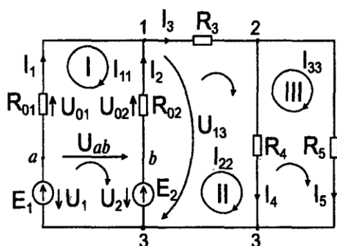
Рисунок 1 – Электрическая цепь
