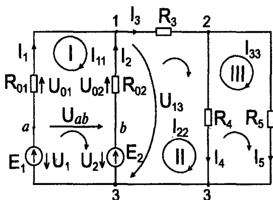
Рисунок 1 – Электрическая цепь
